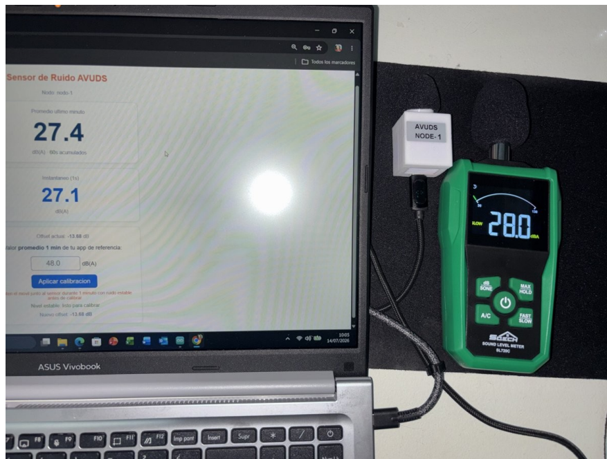
Sensor AVUDS: 27,1 dBA (instantáneo) · SL720C: 28,0 dBA
