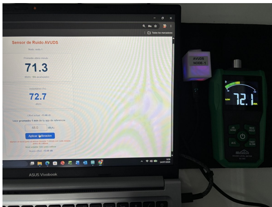
Sensor AVUDS: 72,7 dBA (instantáneo) · SL720C: 72,1 dBA
