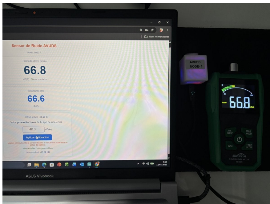
Sensor AVUDS: 66,6 dBA (instantáneo) · SL720C: 66,8 dBA
